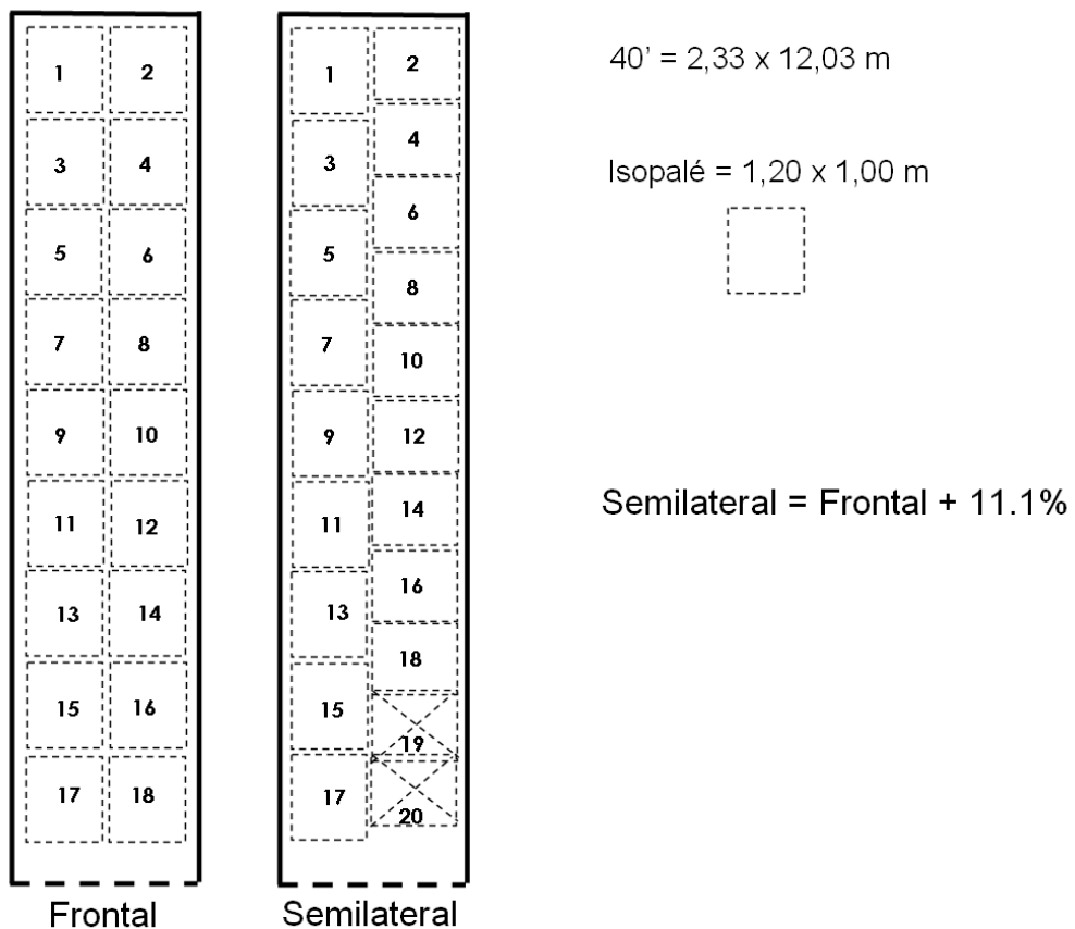
Figura 5: Paletización de un contenedor 40' DV
