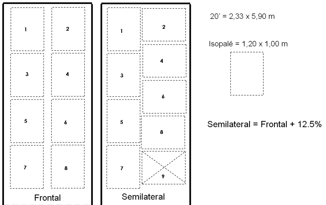
Figura 4: Paletización de un contenedor 20' DV
