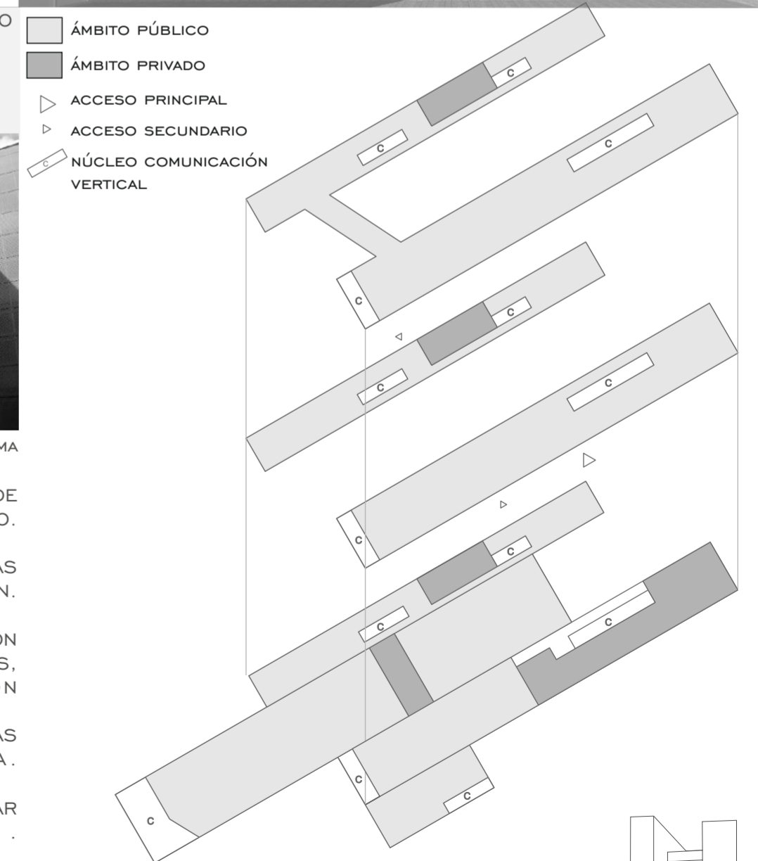
FÁBRICA VAN NELLE - HOLANDA JOHANNES BRINKMAN PALACIO DE LA INDUSTRIA - UCRANIA EMBAJADA DE LOS PAISES BAJOS - BERLIN OMA
