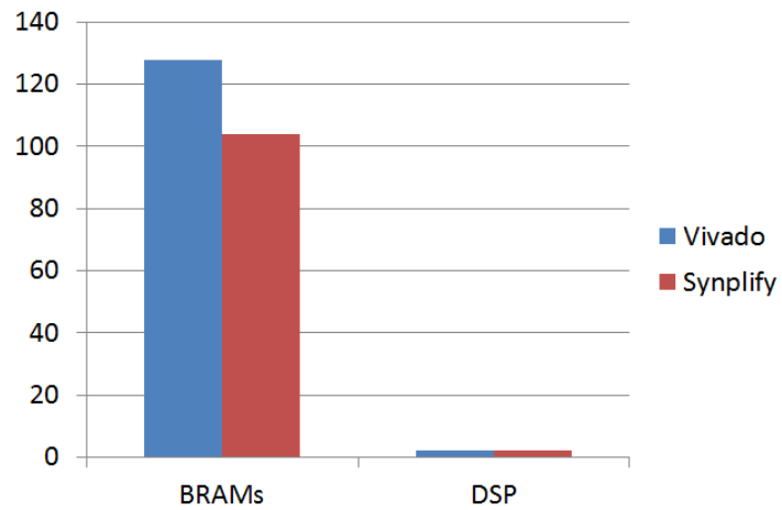
Figura 37. Comparativa BRAM y DSP entre herramientas con top-down
