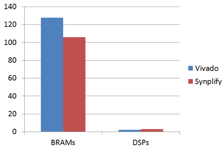
Figura 39. Comparativa BRAM y DSP entre herramientas con bottom-up
