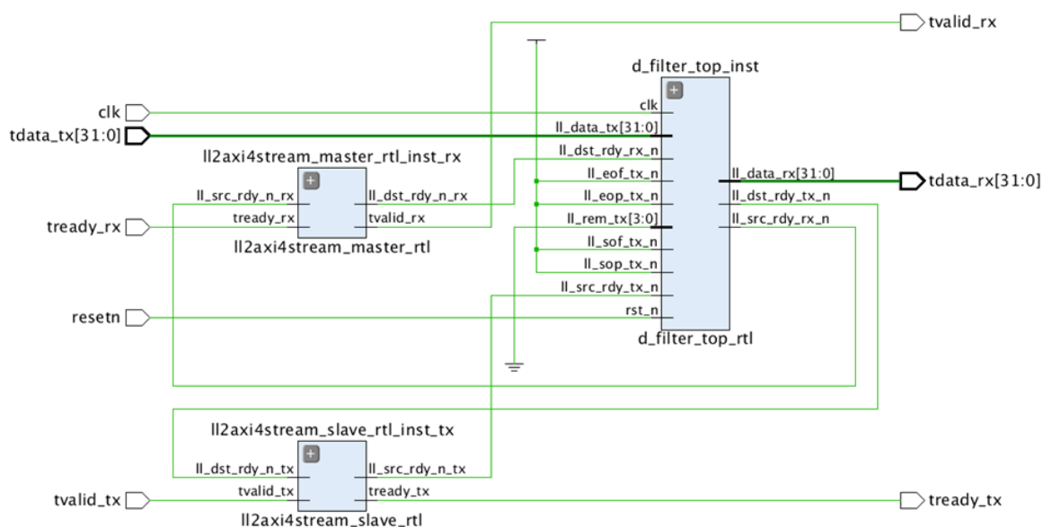
Figura 23. Esquemático RTL
