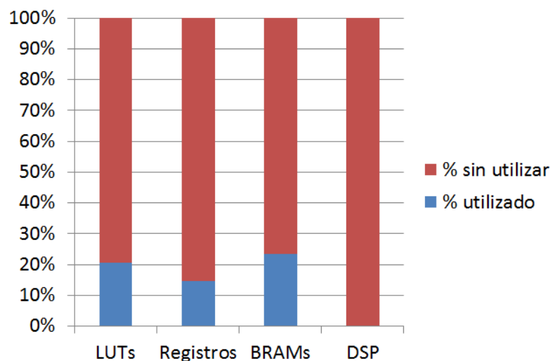
Figura 32. Porcentaje de utilización de recursos
