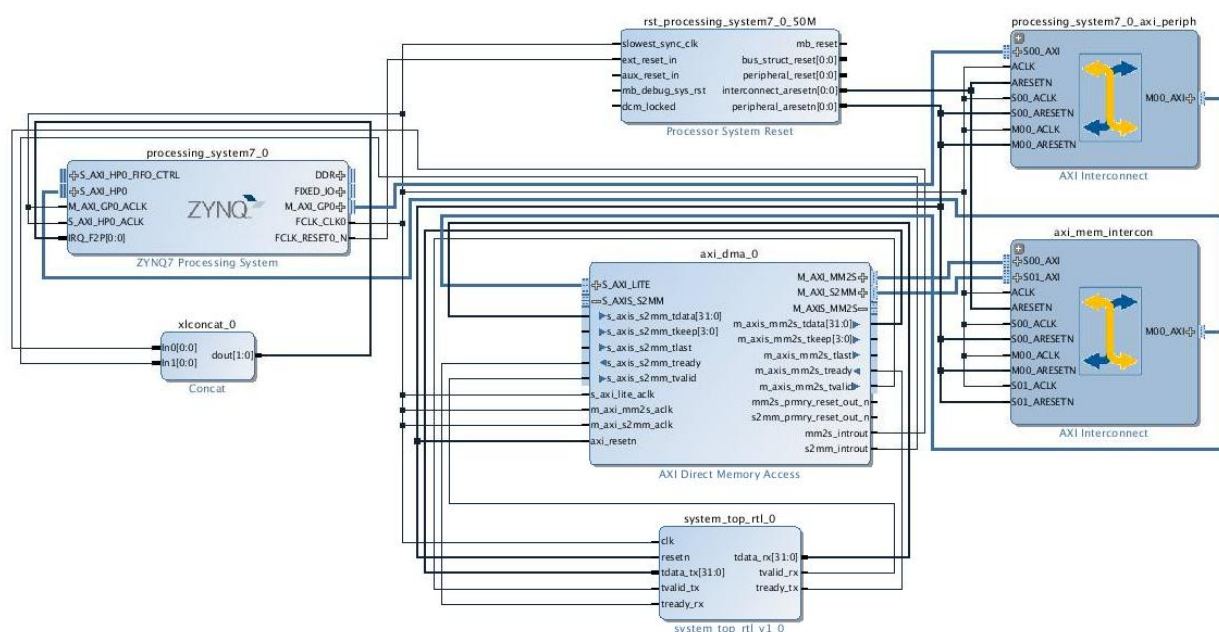
Figura 58. Conexión de todos los bloques IP del sistema
