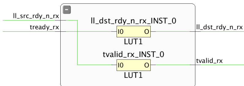
Figura 22. Esquemático del wrapper para recepción
