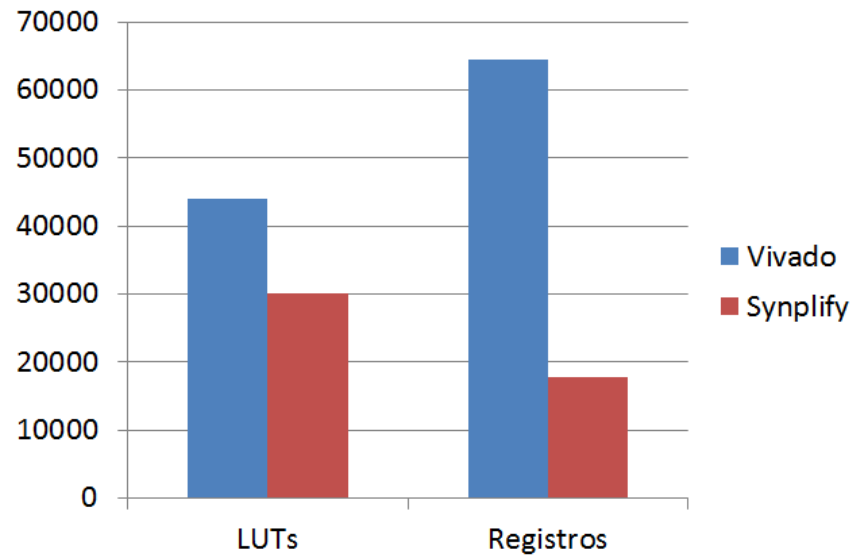
Figura 45. Comparativa LUTs y registros entre herramientas
