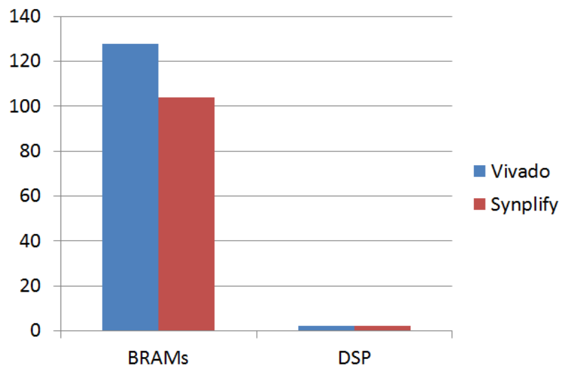
Figura 46. Comparativa BRAMs y DSP entre herramientas
