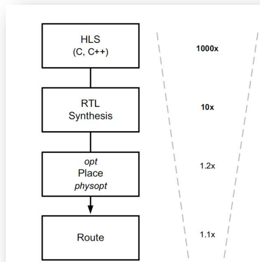
Figura 4. Flujo de diseño Vivado
