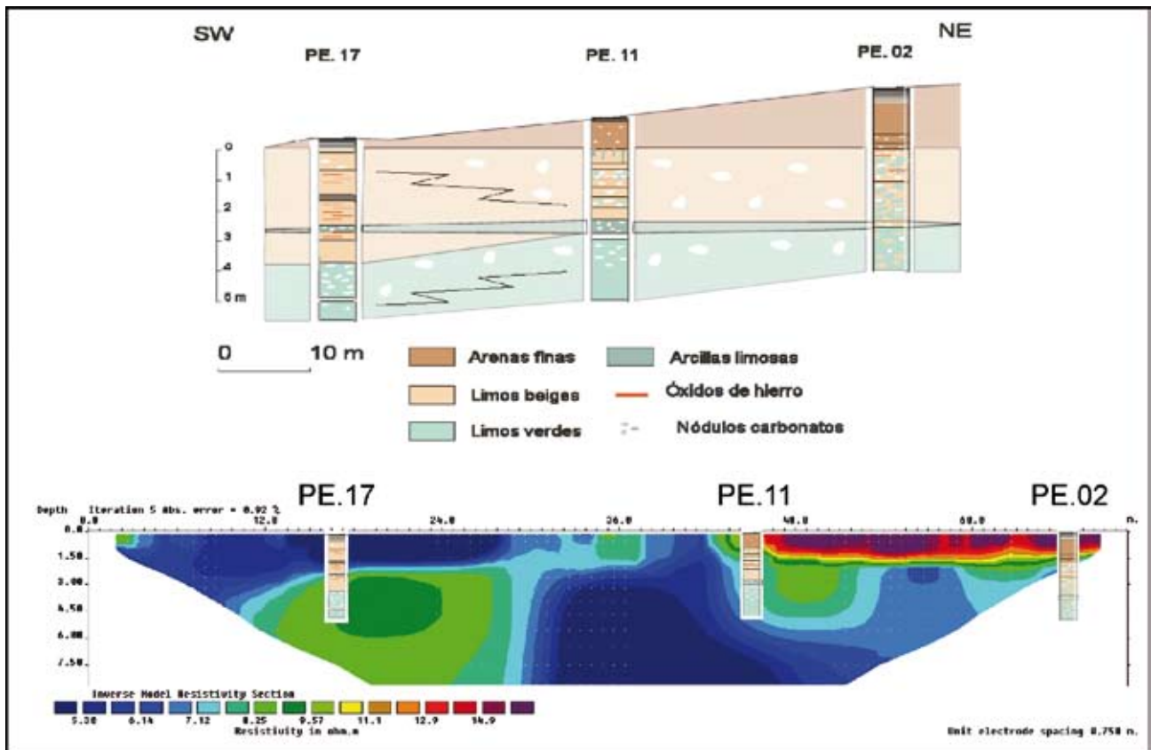
Figura 8. Unidades litológicas y perfil de resistividad obtenidos en la parcela experimental de Carrión de los Céspedes
