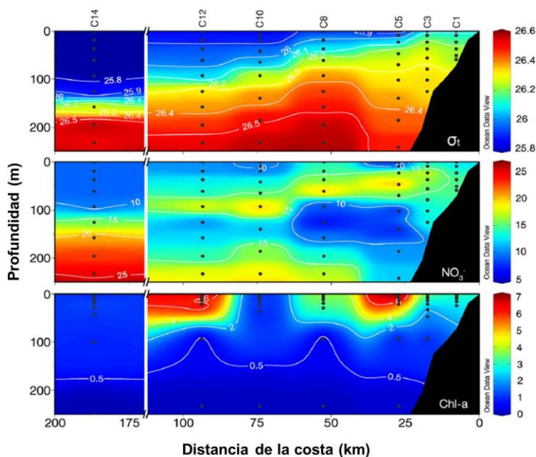
Figura 3 Secciones en profundidad de la densidad potencial ( \sigma_t ), nitratos ( \text{NO}_3^- ) y clorofila ( \text{Chl-a} ) en la sección C de la Figura 1.
