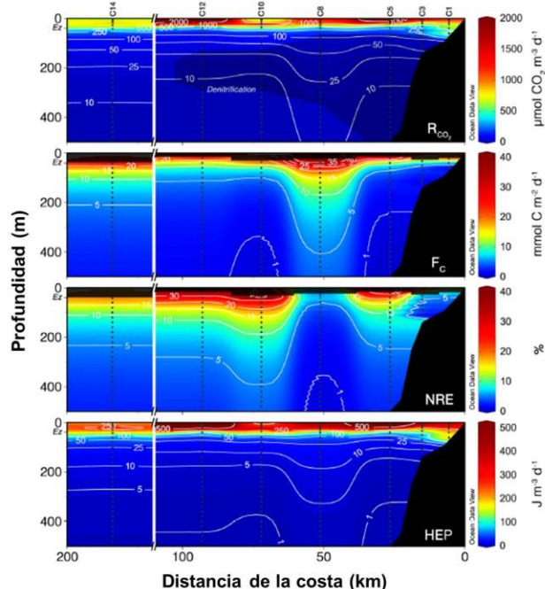
Figura 4 Distribución horizontal del consumo de \text{CO}_2 ( R_{\text{CO}_2} ), Flujo de Carbono ( F_c ), Eficiencia de Retención de Nutrientes (NRE) y Producción de Energía Heterotrófica (HEP) en la sección C de la Figura 1.
