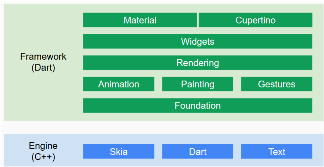
Ilustración 38 Flutter Framework y Engine
