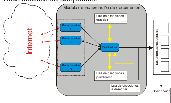
Figura 2: módulo de recuperación de documentos
