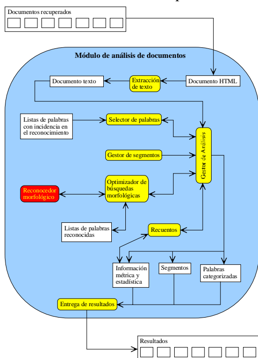
Figura 4: módulo de análisis de documentos
