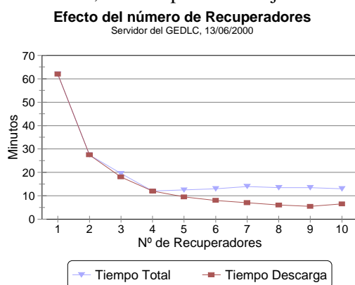
Figura 3: efecto del número de recuperadores
