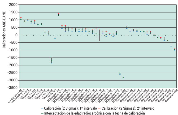
Gráfico I. Seriación de los intervalos de calibración a 2 sigmas (95% de probabilidad) de las fechas C14 obtenidas en contextos arqueológicos protohistóricos de Lanzarote
