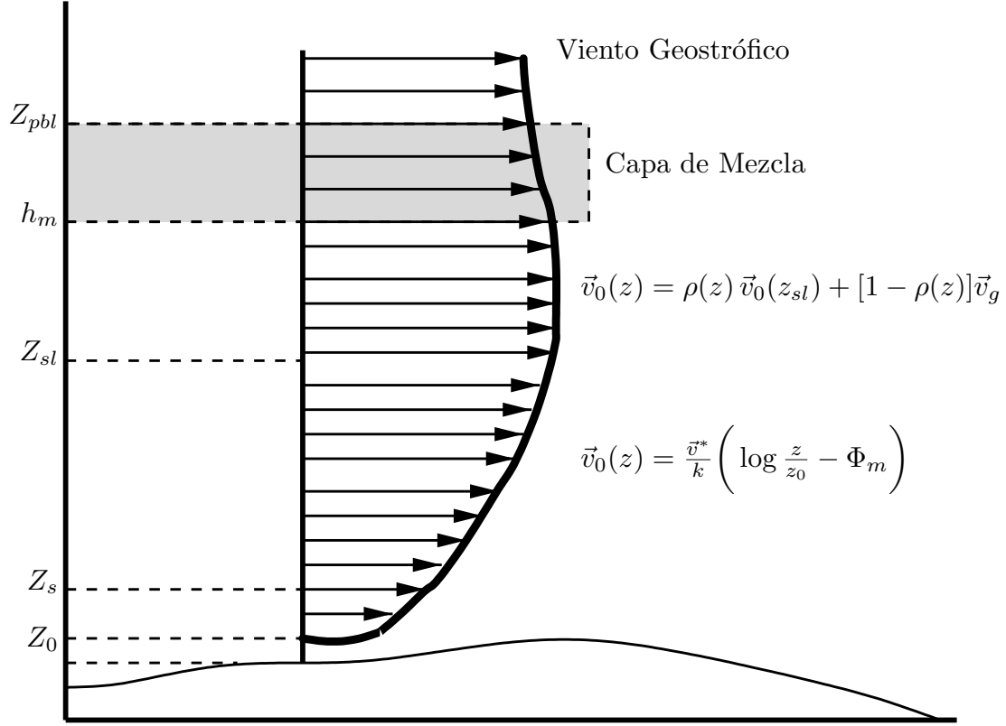
Figura 2.1: Perfil vertical de viento definido sobre cada capa de la estratificación atmosférica.
