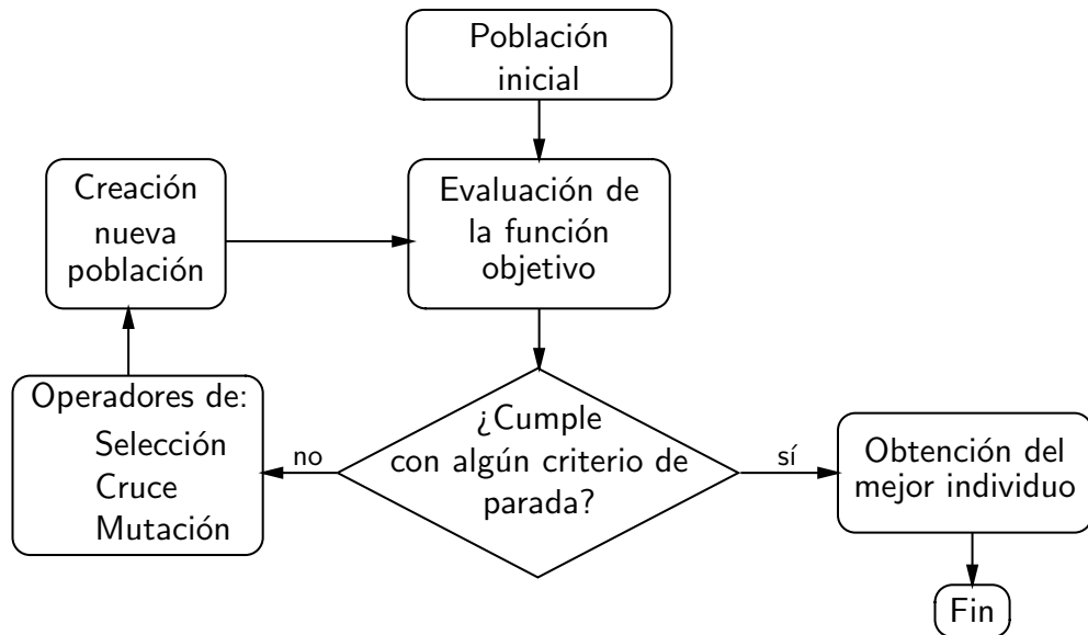
Figura 4.1: Diagrama del funcionamiento de los AG
