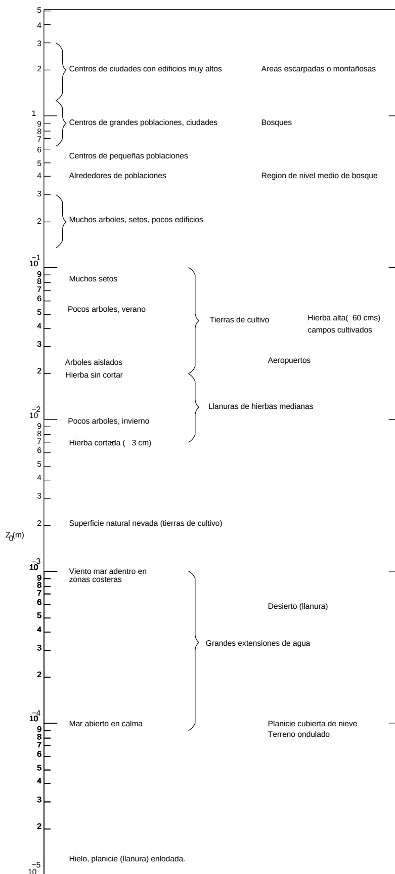
Figura 2.2: Longitud de rugosidad: valores aproximados de z_0 para distintos tipos de terreno definidos por McRae (1982)
