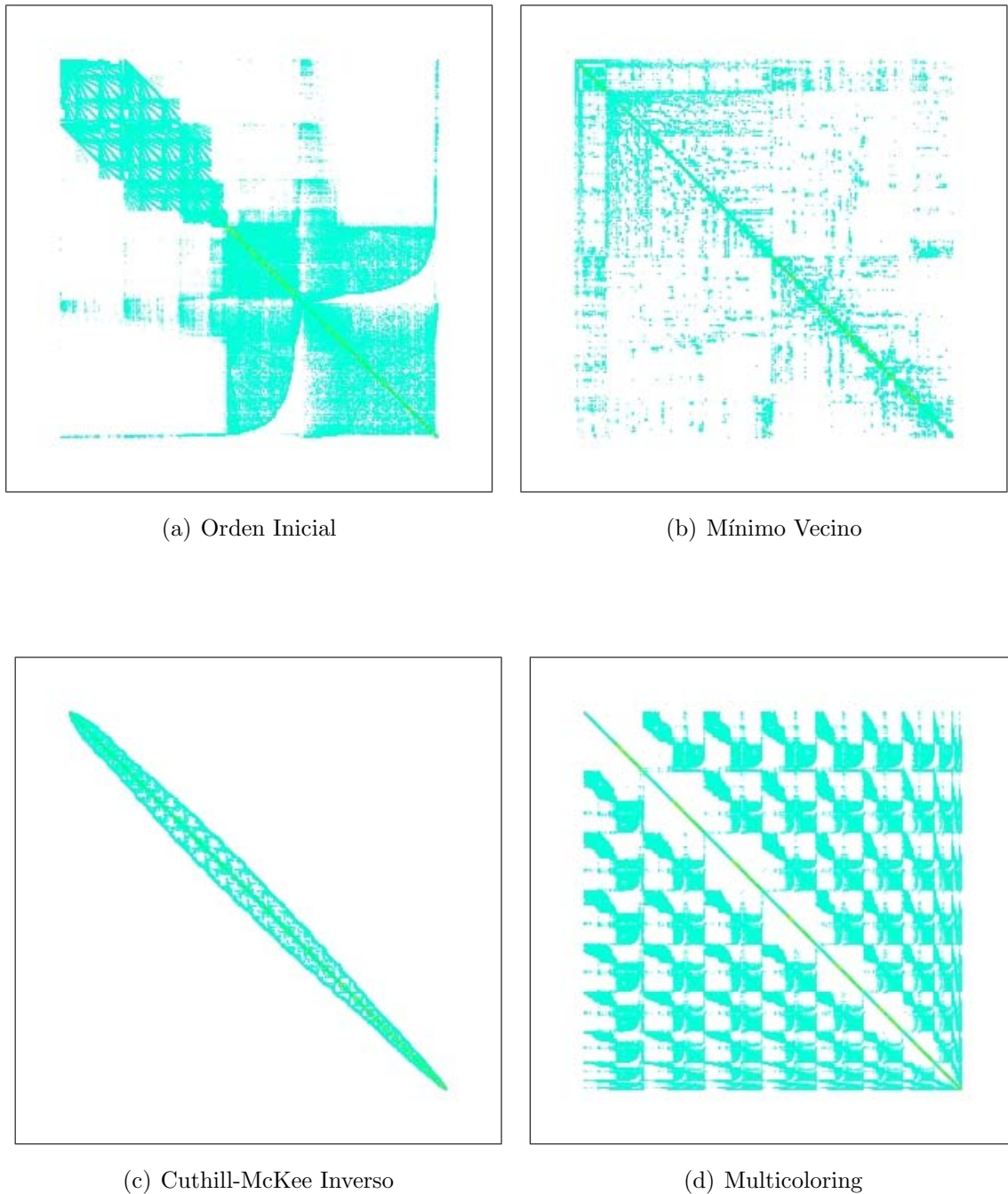
Figura 9.1: Patrones de ‘sparsidad’ de las matrices, con su orden inicial y una vez reordenadas
