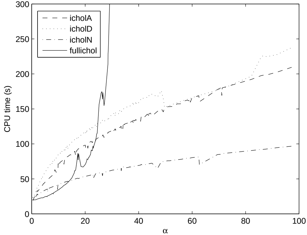
Figura 9.3: Campo de Viento de 98.999 ecuaciones: Convergencia del Gradiente Conjugado Precondicionado, con varios Precondicionadores ICHOL, para diferentes valores del parámetro \alpha , elegidos usando una distribución normal
