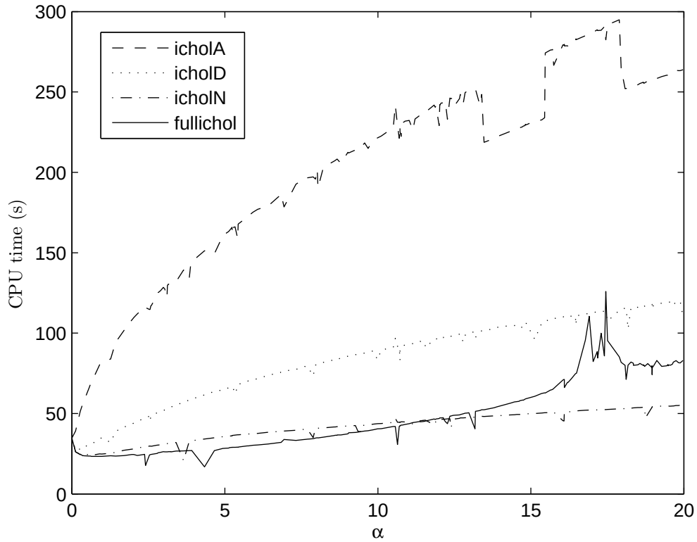
Figura 9.2: Campo de Viento de 98.999 ecuaciones: Convergencia del Gradiente Conjugado Precondicionado, con varios Precondicionadores ICHOL, para diferentes valores del parámetro \alpha , aleatoriamente calculados
