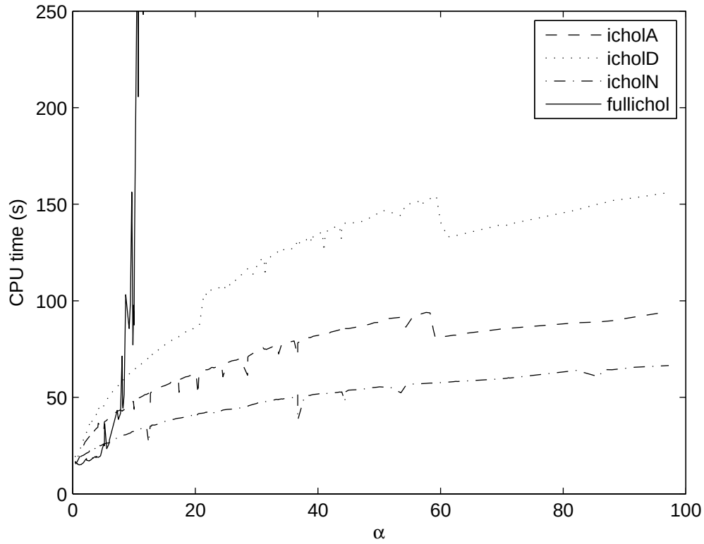
Figura 9.5: Campo de Viento de 100.643 ecuaciones: Convergencia del Gradiente Conjugado Precondicionado, con varios Precondicionadores ICHOL, para diferentes valores del parámetro \alpha , elegidos usando una distribución normal
