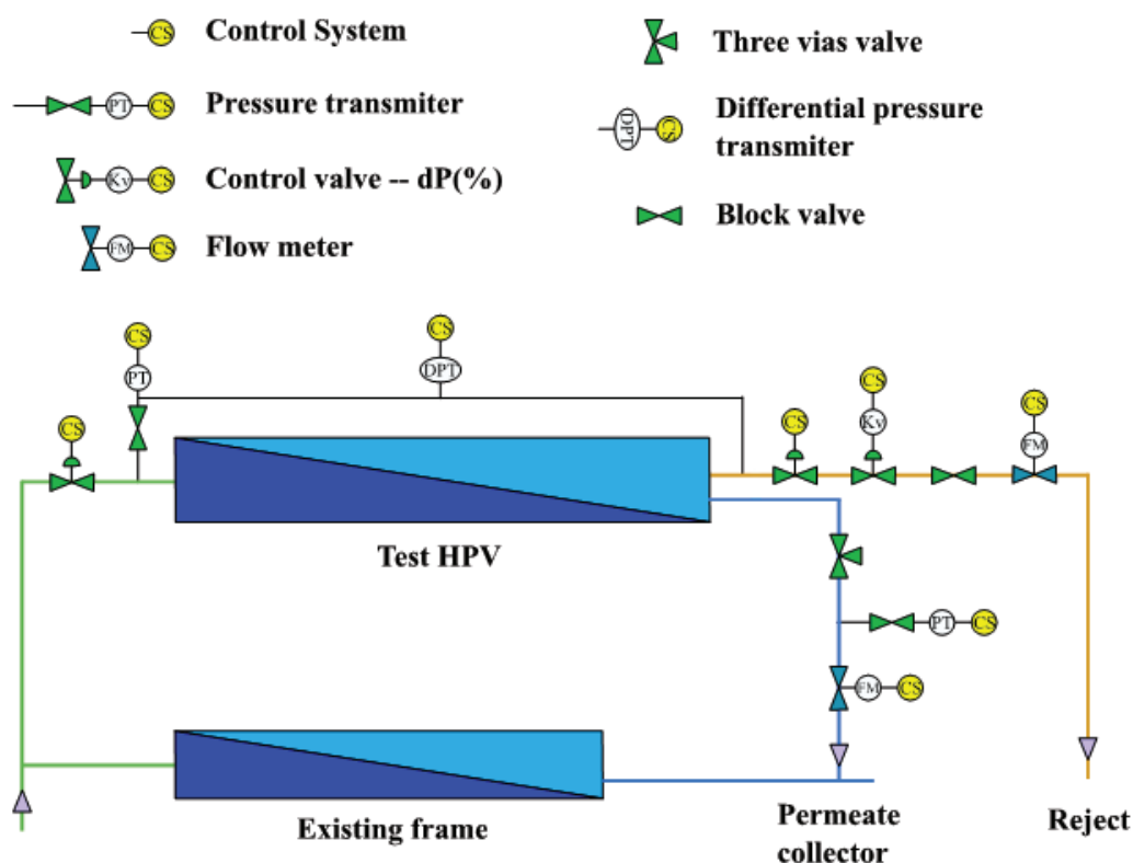
Fig. 3. Test HPV diagram.
