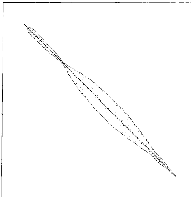
Figura 10.63: Estructura sparse de la matriz convdifhor para n = 13190 reordenada con Cuthill-McKee Inverso
