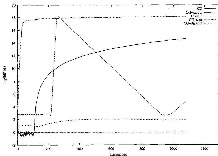
Figura 10.8: Convergencia del CG con distintos preconditionadores para SHERMAN2
