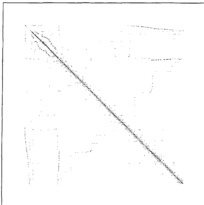
Figura 10.57: Estructura sparse de la matriz convdifhor para n = 3423 reordenada con Mínimo Vecino
