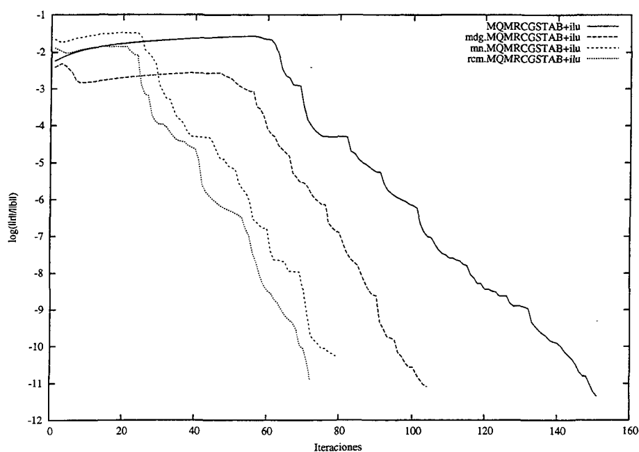
Figura 10.60: Efecto de la reordenación en la convergencia del QMRCGSTAB precondicionado con ILU(0) para convdifhor (3423 ecuaciones)
