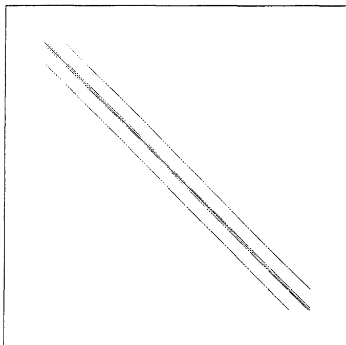
Figura 10.10: Estructura sparse de la matriz SHERMAN3
