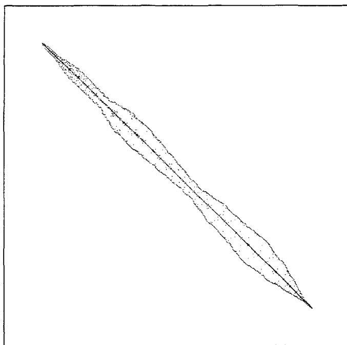
Figura 10.58: Estructura sparse de la matriz convdifhor para n = 3423 reordenada con Cuthill-McKee Inverso
