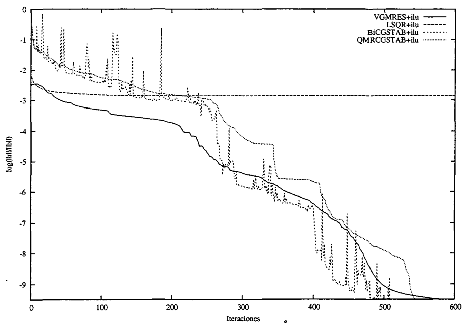
Figura 10.64: Convergencia de distintos métodos de Krylov preconditionados con ILU(0) para convdifhor (13190 ecuaciones)
