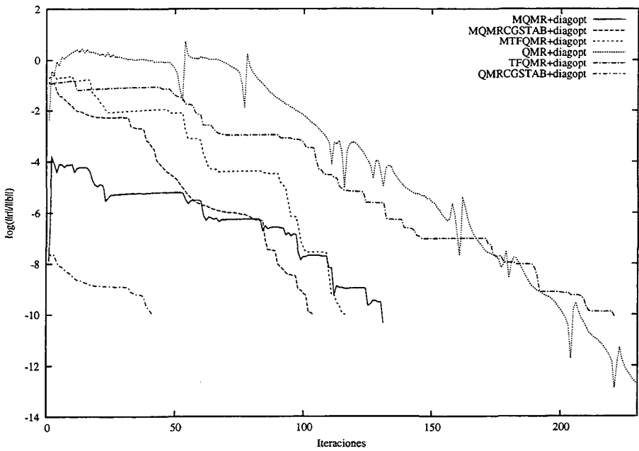
Figura 10.46: Convergencia de distintos métodos tipo QMR con preconditionador Diagonal Óptimo para WATT1
