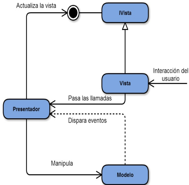
Figura 2.1: Diagrama de la arquitectura Modelo-Vista-Presentador
