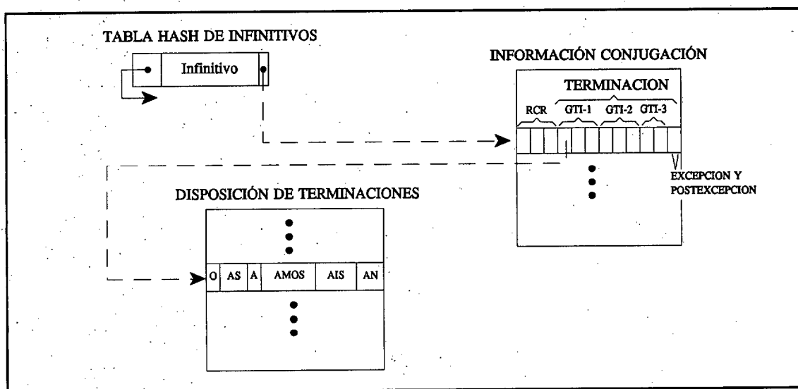
Figura 5: Estructura de Conjugación
