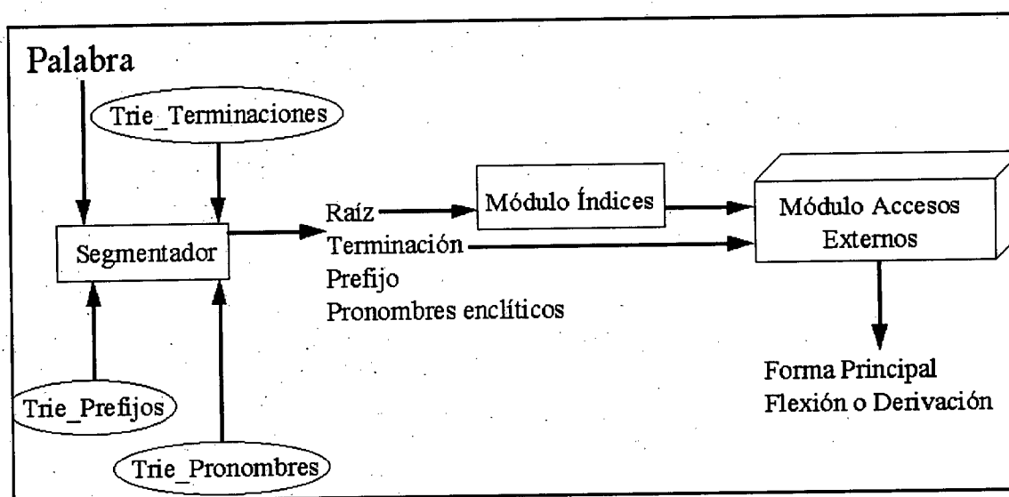
Figura 4: Esquema del Reconocedor
