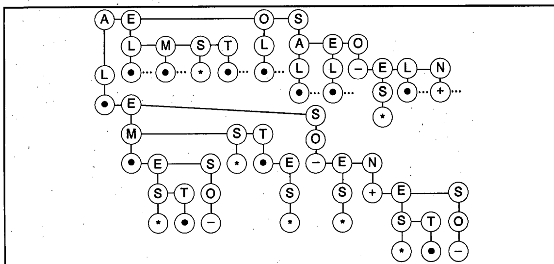
Figura 6: Trie de pronombres enclíticos
