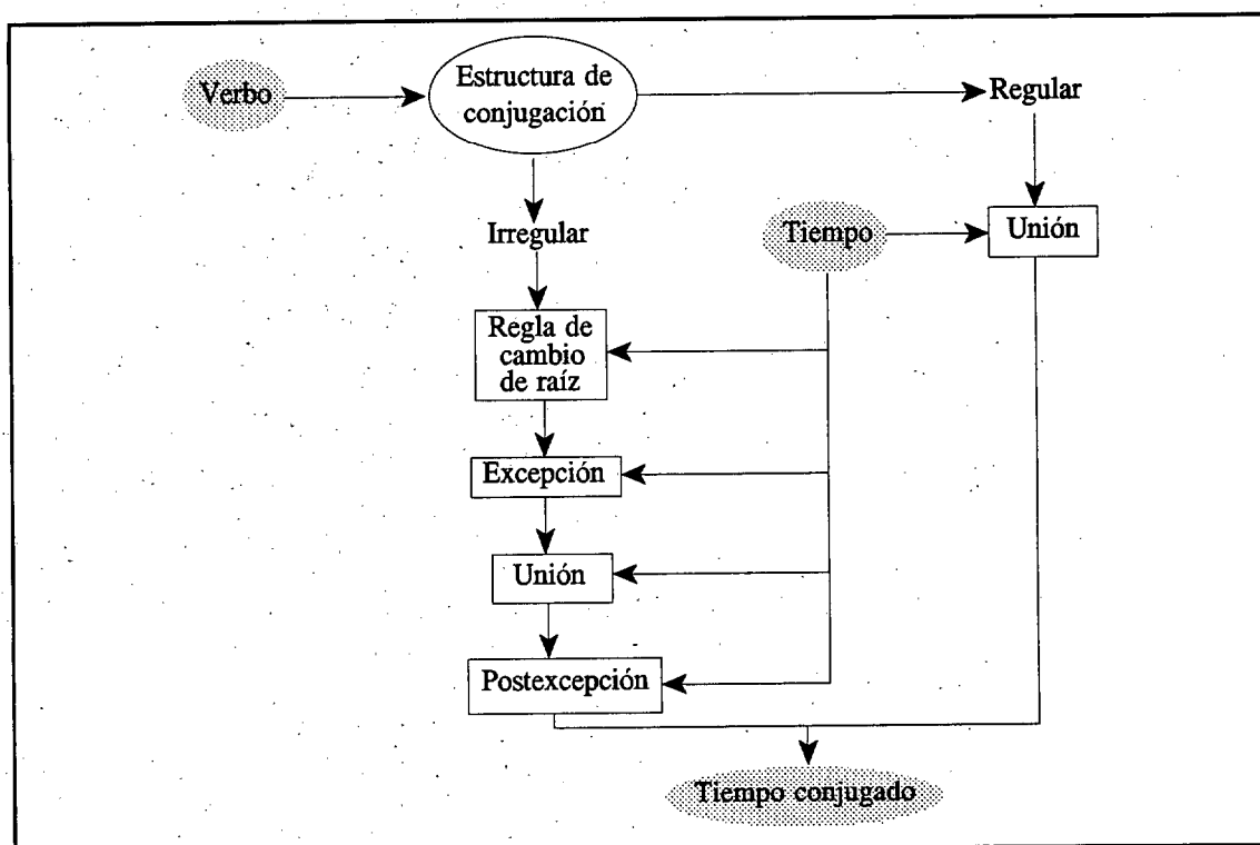
Figura 6: Proceso de conjugación
