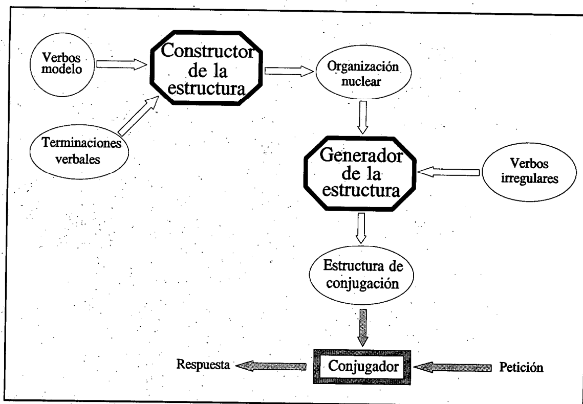
Figura 4: Desarrollo del Conjugador
