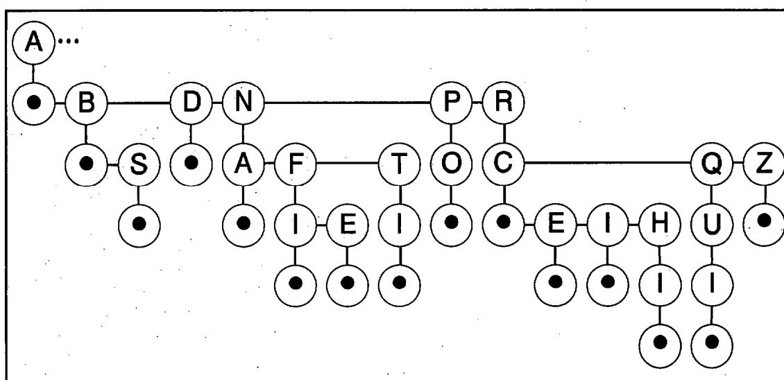
Figura 5: Trie de prefijos
