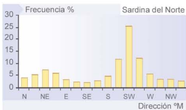
Figura 19. Diagrama de distribución de la dirección de la corriente en Sardina del Norte, desde diciembre de 1999 hasta noviembre de 2000.
