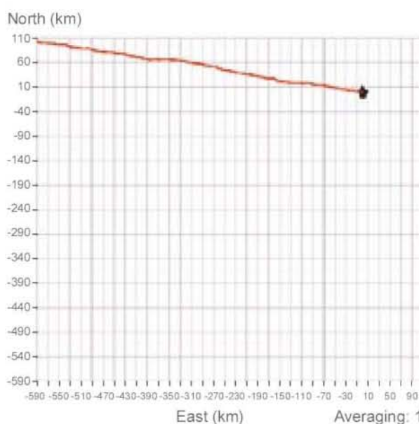
Figura 25. Diagrama del vector progresivo de la corriente en Arguineguín, desde abril a diciembre de 2001.
