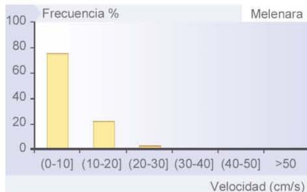
Figura 20. Diagrama de distribución de la velocidad de la corriente en Melenara, desde junio a septiembre de 2001.
