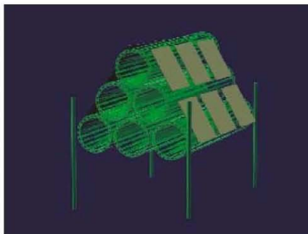
Figura 16. Diseño original de los arrecifes.
