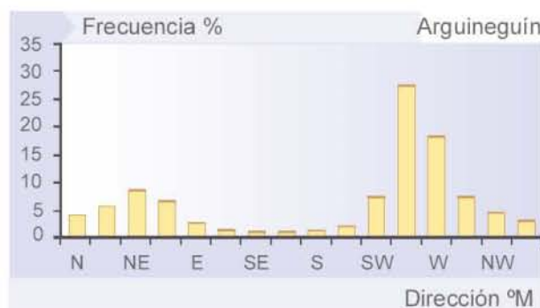
Figura 24. Diagrama de distribución de la dirección de la corriente en Arguineguín, desde abril a diciembre de 2000.
