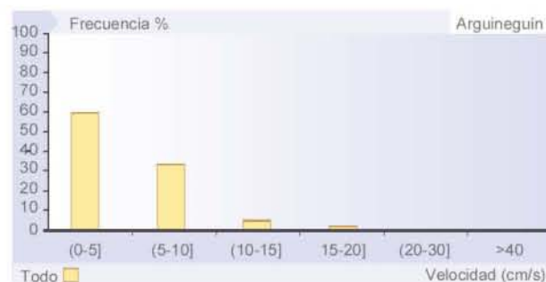
Figura 23. Diagrama de distribución de la velocidad de la corriente en Arguineguín, desde abril a diciembre de 2000.
