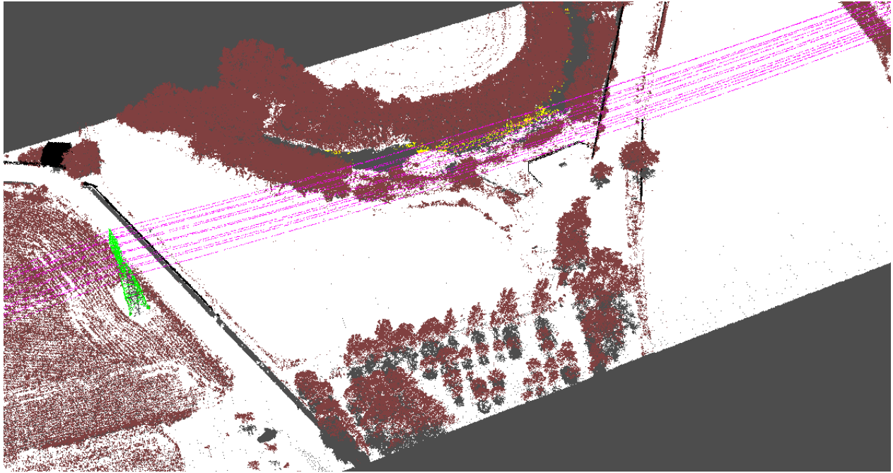
Ilustración 4.23: Segmento de una escena de ECLAIR
