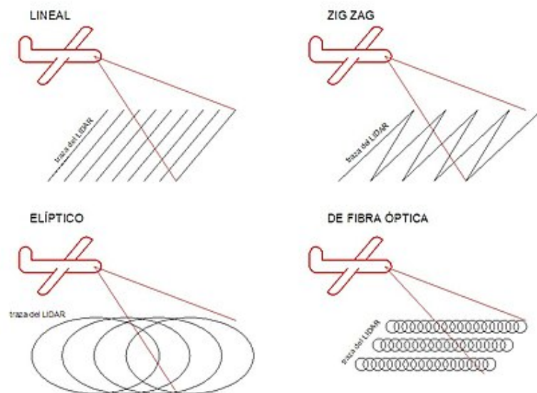
Ilustración 2.2: Esquema de los cuatro grandes tipos de LiDAR Aéreo
