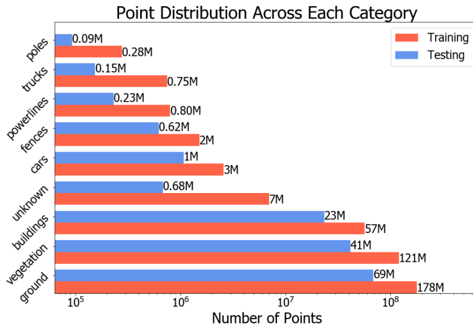
Ilustración 3.5: Distribución de clases dataset DALES. Cortesía de la University of Dayton
