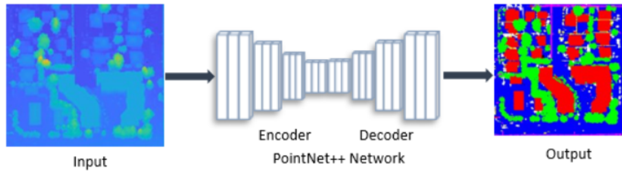
Ilustración 2.15: Abstracción del funcionamiento de la Pointnet++. Cortesía de MatLab
