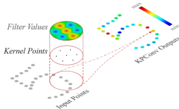
Ilustración 2.11: Abstracción del funcionamiento de KPConv. Cortesía de Mines Paris Tech, Facebook AI Research y Stanford University
