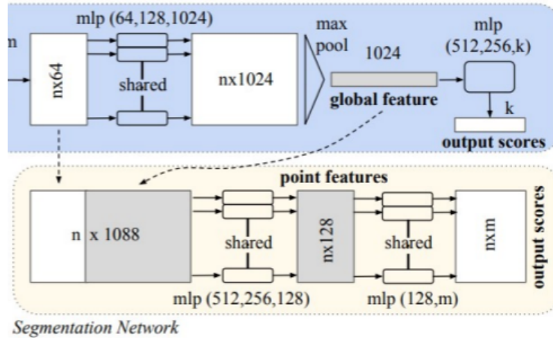
Ilustración 2.10: Ampliación de la red de clasificación para la segmentación
