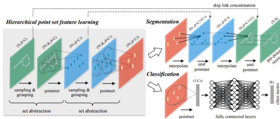
Ilustración 2.16: Detalle de la estructura de la Pointnet++. Cortesía de Stanford University
