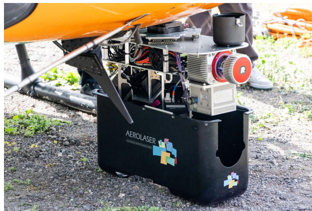
Ilustración 3.9: Sensor LiDAR propiedad de AeroLaser System S.L.
