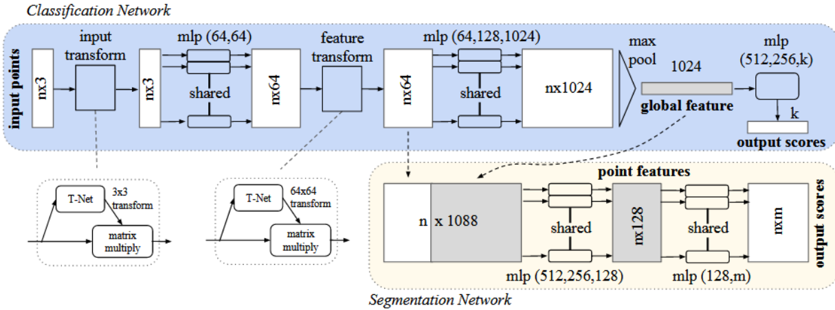
Ilustración 2.7: Arquitectura general de la Pointnet. Imagen cortesía de la universidad de Stanford
