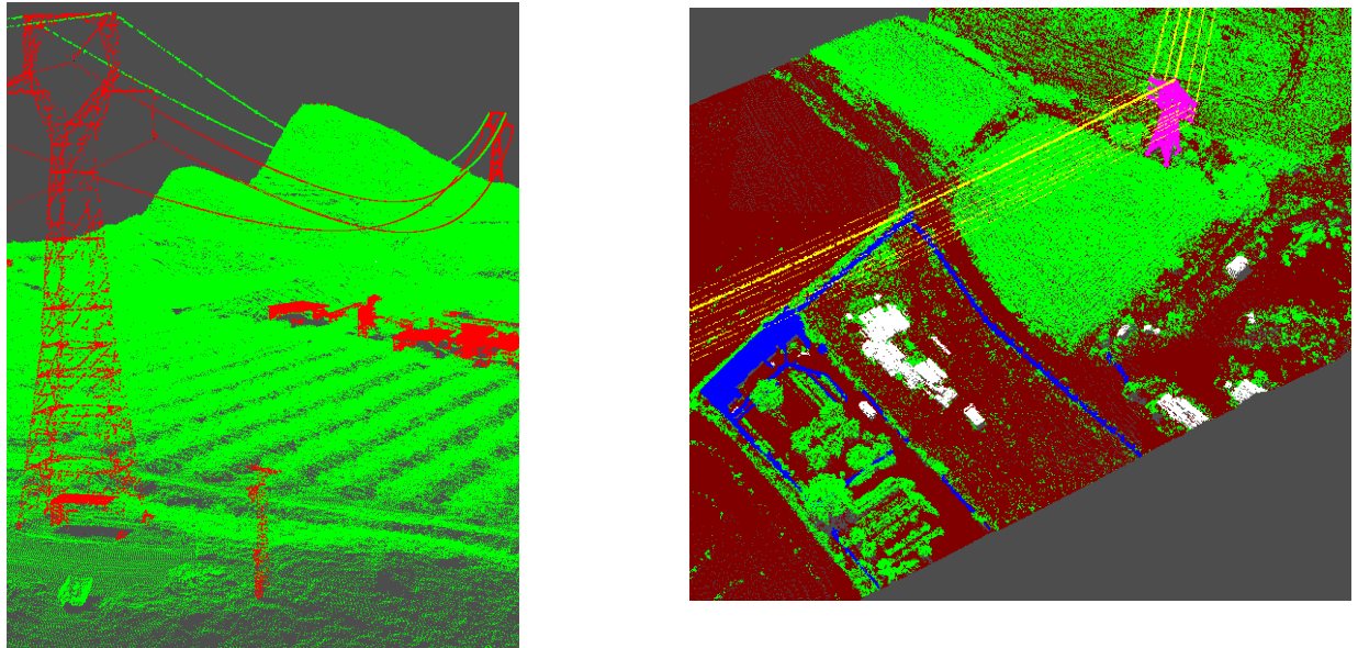
Ilustración 4.14: Comparativa entre ground truth y aciertos/fallos antes del transfer learning
