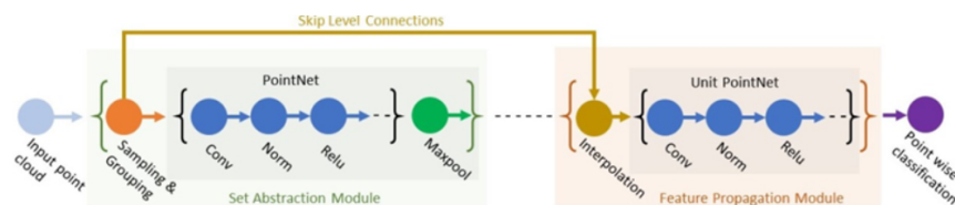
Ilustración 2.17: Estructura general de la segmentación semántica con Pointnet++. Cortesía de MatLab
