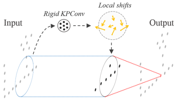
Ilustración 2.14: Representación gráfica de los Kernels deformables. Cortesía de Mines Paris Tech, Facebook AI Research y Stanford University
