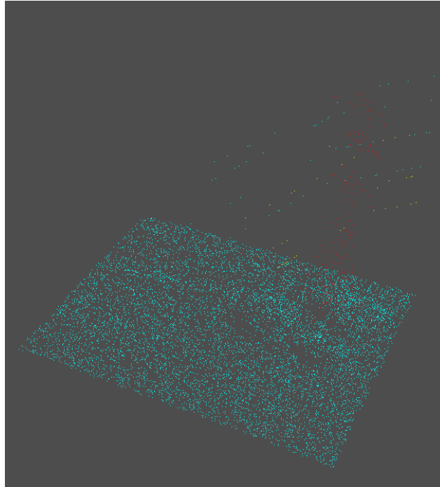
Ilustración 4.17: Segmentación de una celda de AeroLaser. Se puede apreciar cómo buena parte de los cables se clasifican como terreno
