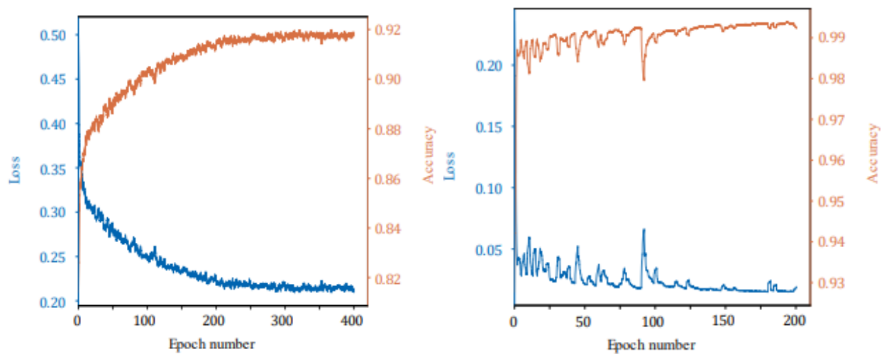
Ilustración 2.19: Relación entre Loss y Accuracy en el entrenamiento de KPConv TL (izq) y KPConv R (der)
