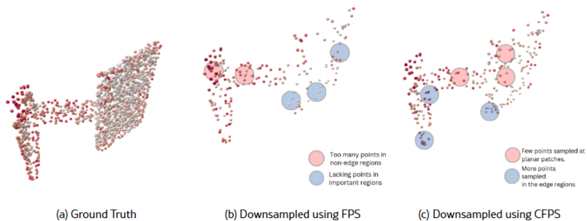
Ilustración 5.2: Comparativa entre FPS y CFPS en geometrías irregulares. Cortesía de la University of Texas at Austin
