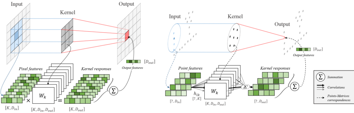
Ilustración 2.13: Comparativa entre clasificación de imágenes tradicional y KPConv. Cortesía de Mines Paris Tech, Facebook AI Research y Stanford University
