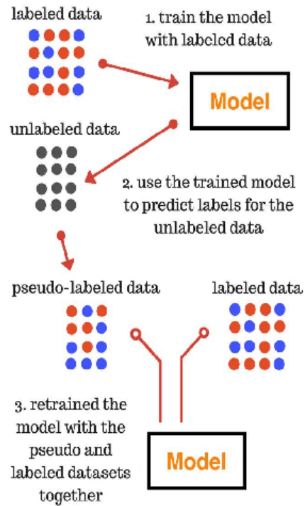
Ilustración 3.8: Esquema de funcionamiento del pseudolabeling. Cortesía de Medium
