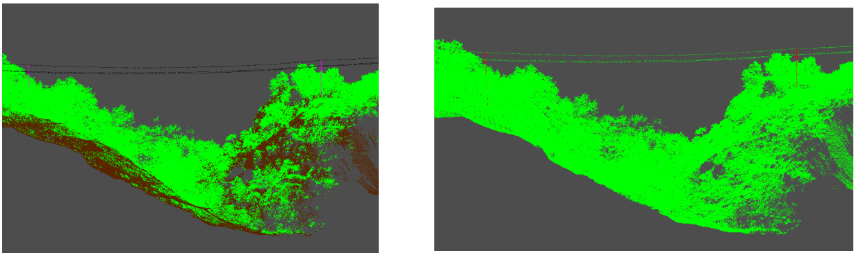
Ilustración 4.20: Comparativa entre ground truth y aciertos/fallos. Los fallos en rojo, los aciertos en verde
