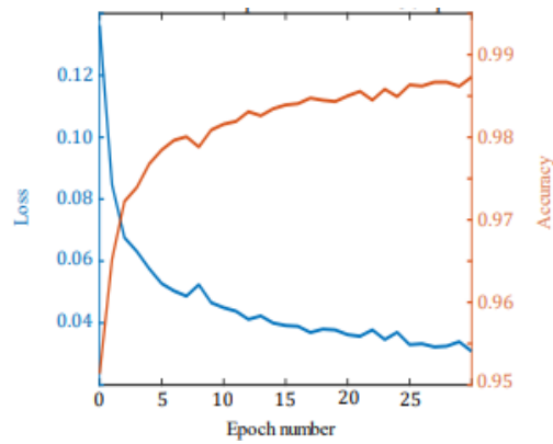
Ilustración 2.18: Relación entre Loss y Accuracy en el entrenamiento de la Pointnet. Cortesía de la Universidade de Vigo
