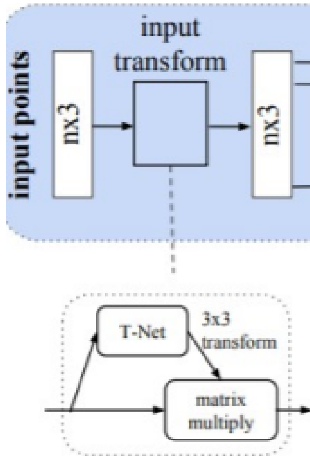
Ilustración 2.8: Entrada y transformación de la entrada
