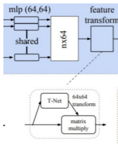
Ilustración 2.9: Perceptrón multicapa (MLP) y modificación de la salida
