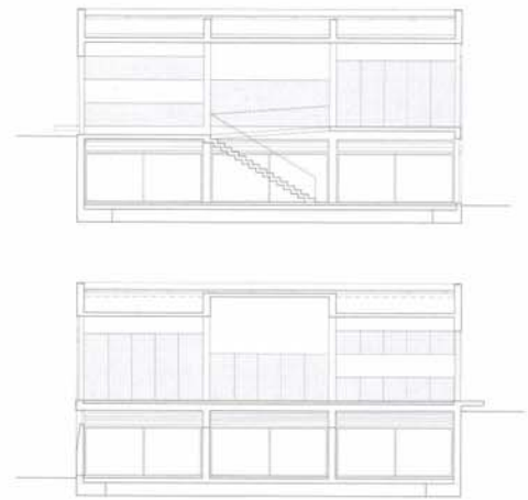
Längsschnitte Longitudinal sections 1:333
