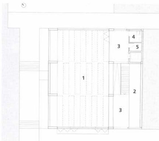
Oberes Geschoss Upper floor 1:333
