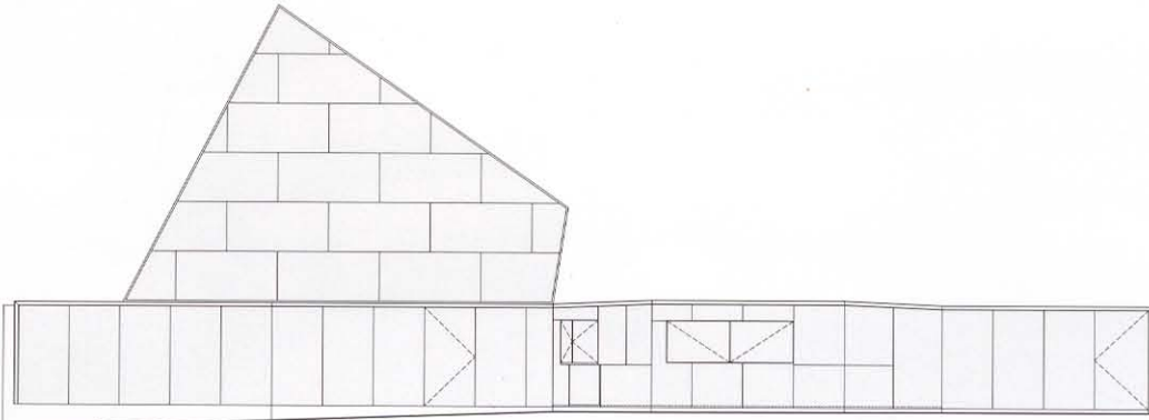
Quiosco. Piel. Desplegado de paneles fenólicos Drink stand. Skin. True dimension panels
