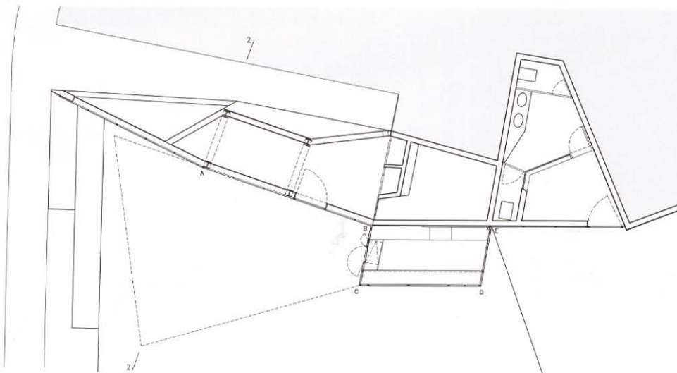
Planta del Quiosco Drink stand plan
