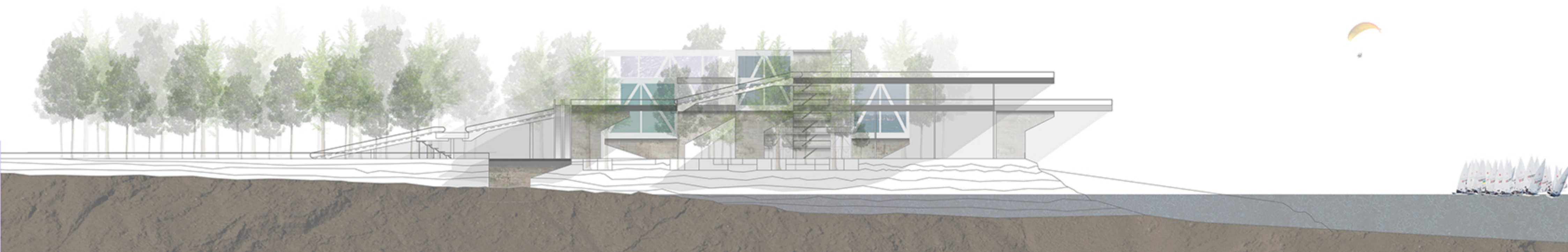
ALZADO OESTE.
