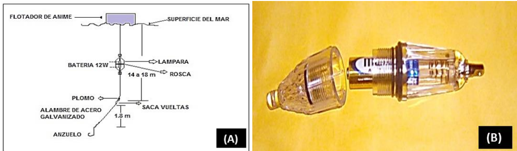
Figura 3. (A) Esquema del sistema de pesca con cordel y dispositivo eléctrico que emite luz. (B) Fotografía del dispositivo eléctrico que emite luz y atrae los peces (Tajalí).
