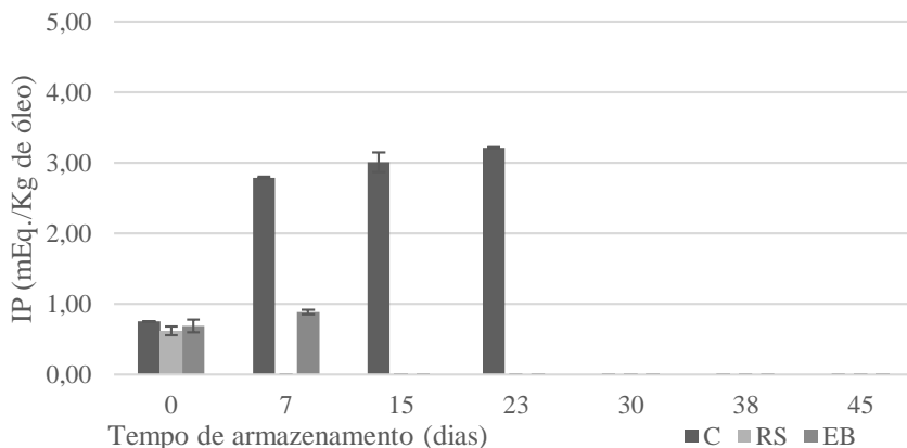
Figura 8. Variações do índice de peróxidos ao longo do tempo de armazenamento para as três formulações em estudadas: C - Controle, RS - Redução de Sal e EB - Extrato Bioativo. Valores médios \pm desvio padrão de três réplicas. Barras verticais indicam intervalos de confiança de 0,95.
