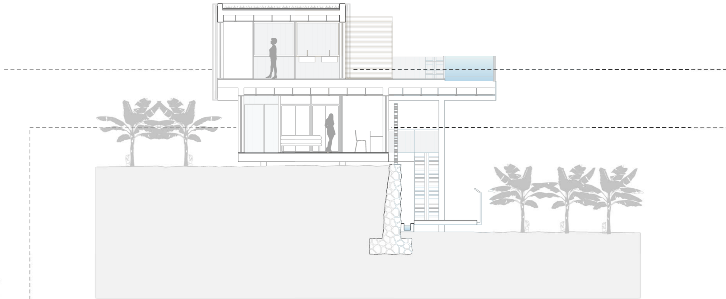
SECCION TRANSVERSAL E 1/100
