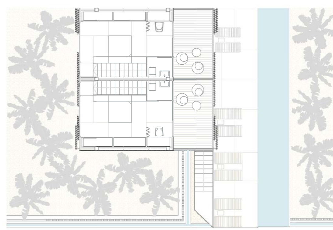
PLANTA SEGUNDA. DORMITORIO + TERRAZA E 1/150
