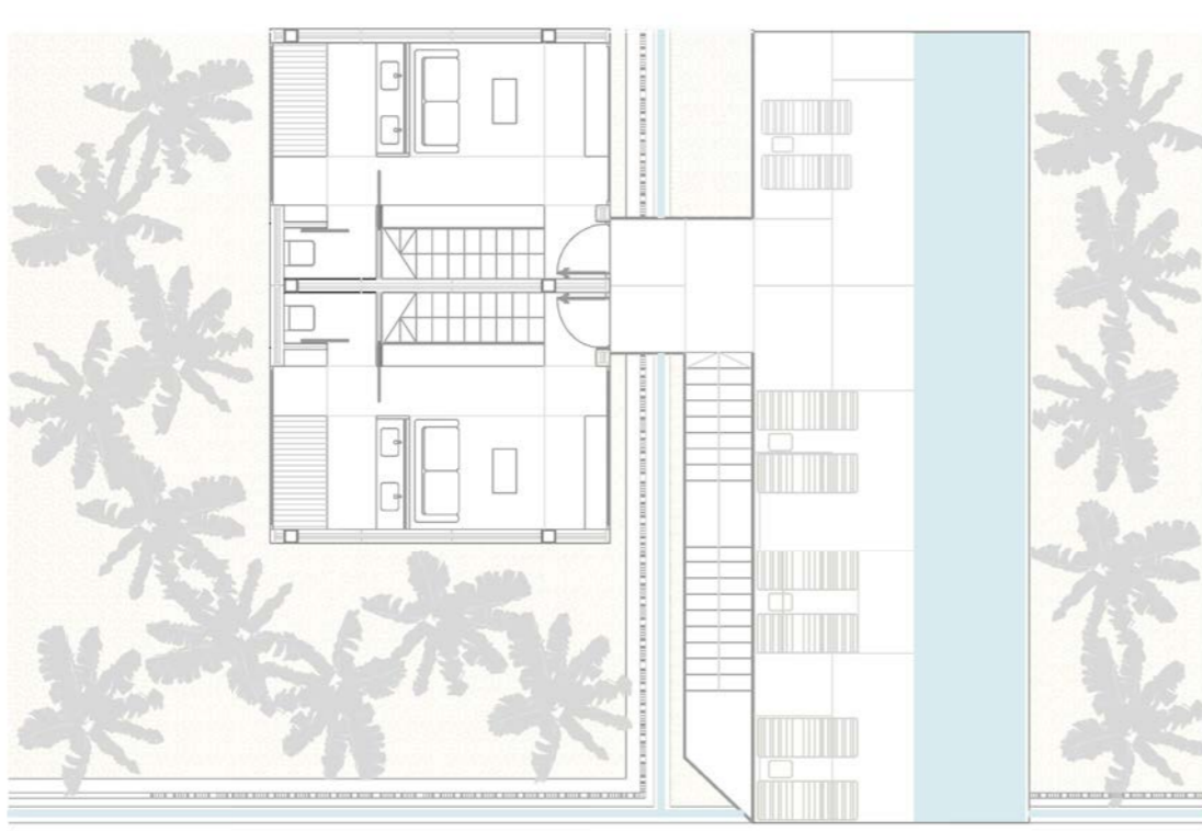
PLANTA PRIMERA. SALÓN E 1/150
