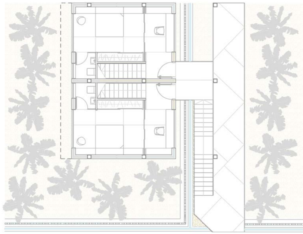
PLANTA PRIMERA. DORMITORIO E 1/150
