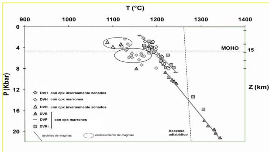
Fig. 2. Correlación entre la P y T de cristalización de los cpx marrones y cpx inversamente zonados utilizando el termobarómetro de Putirka et al. (2003). Modificado de Aulinas (2008).
