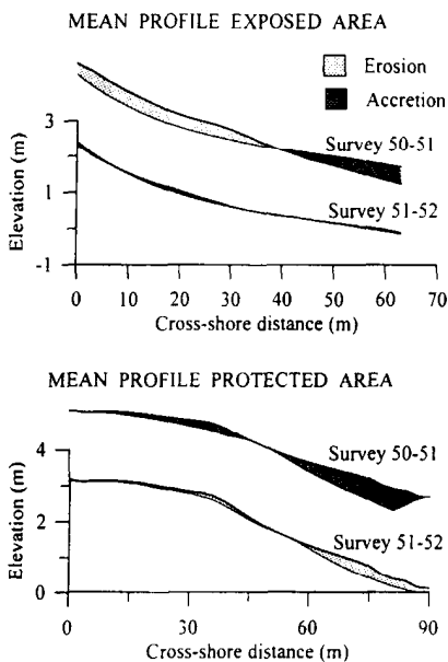
Fig. 4.- Cambios en el perfil de playa inducidos por el temporal de febrero de 1991.
