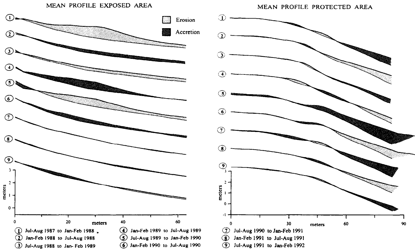
Fig. 2.- Cambios estacionales para perfiles medios de las zonas expuesta y resguardada
